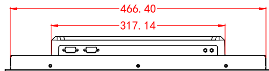
外嵌式QG-185WL尺寸图（全铝款）
