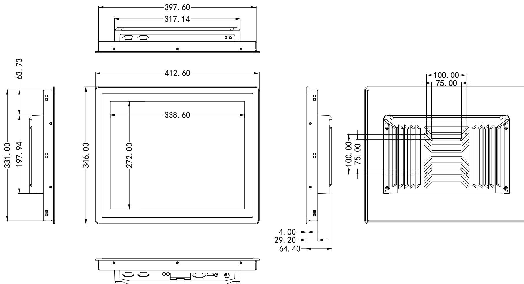
外嵌式QG-170WL尺寸图（全铝款）
