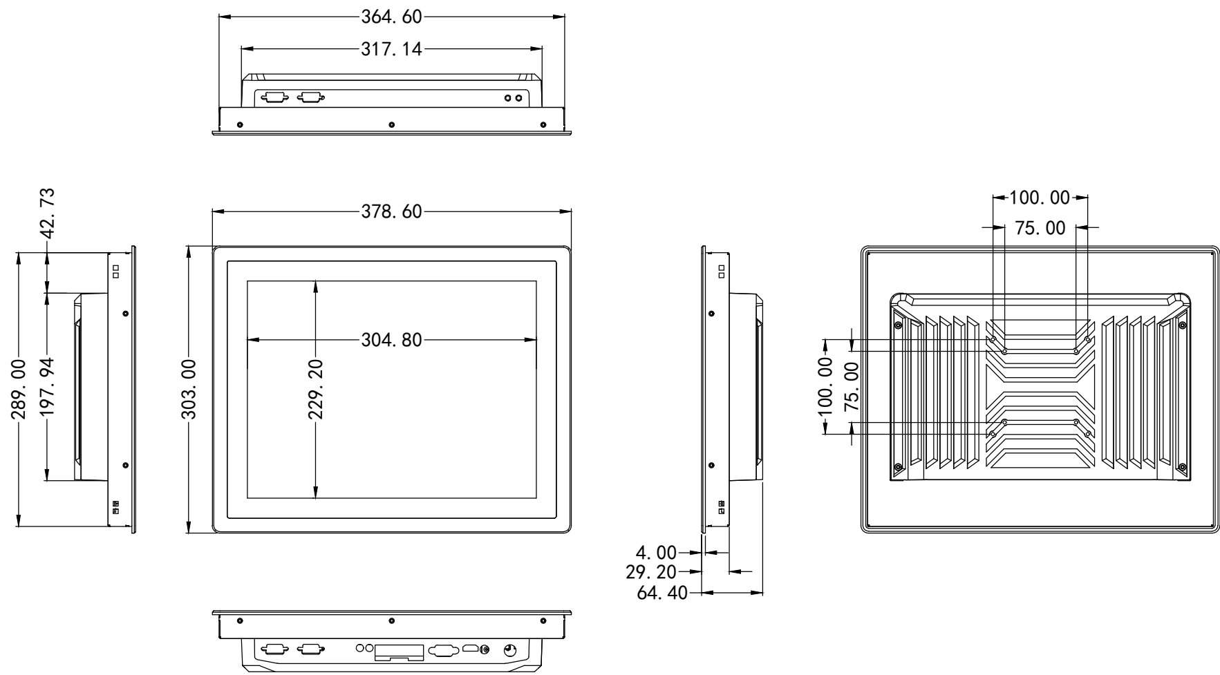
外嵌式QG-150WL尺寸图（全铝款）
