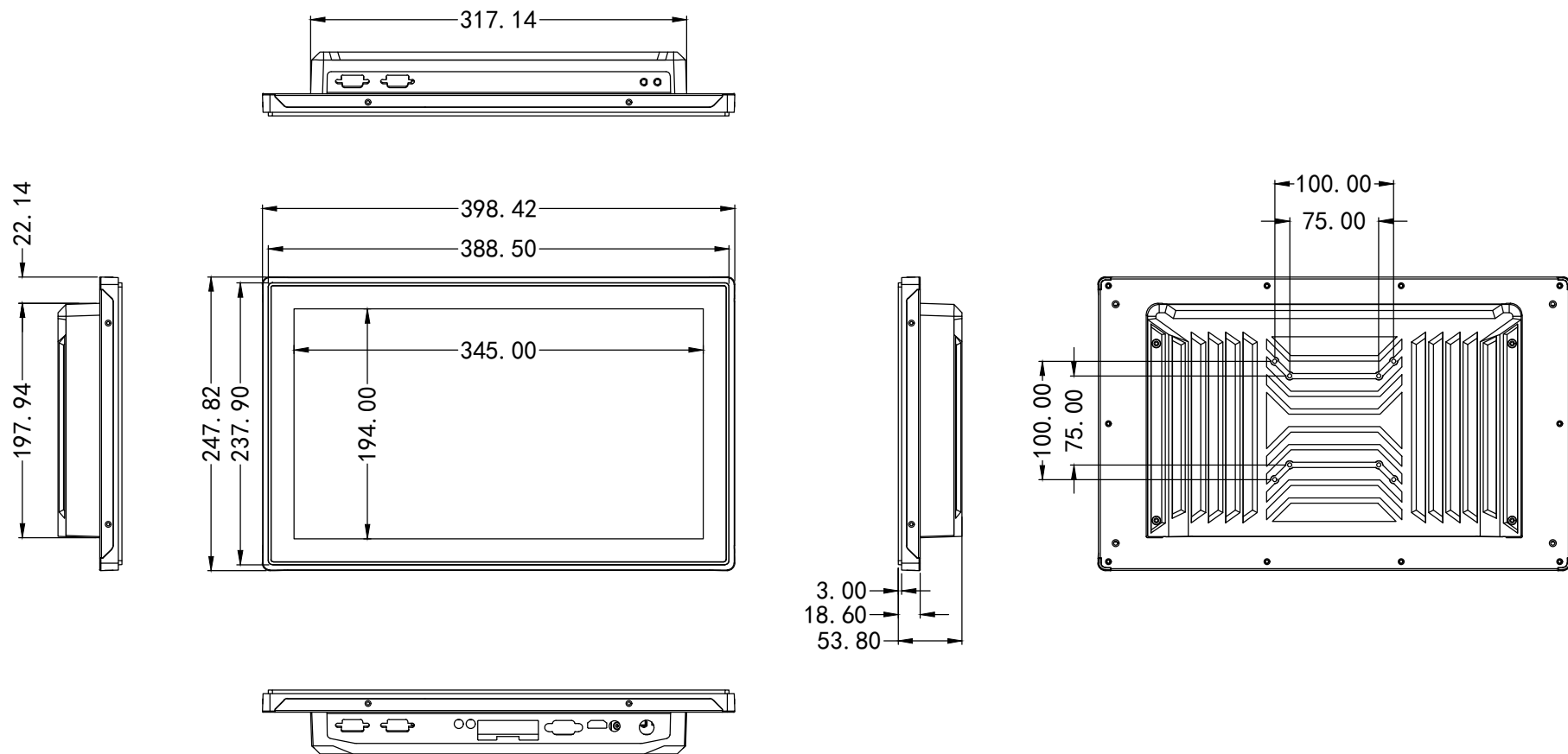
内嵌式QG-156NL尺寸图（全铝款）
